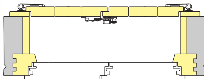
Contraventana con antepecho (mocheta) revestida de madera
