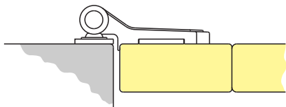
Cierre enrasado
